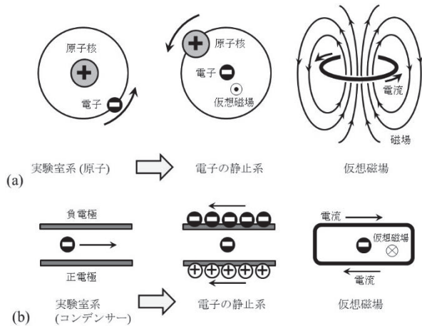
図6 スピン軌道相互作用のもとになる仮想磁場
